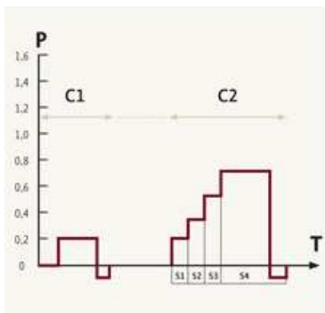
« Sequential » program
